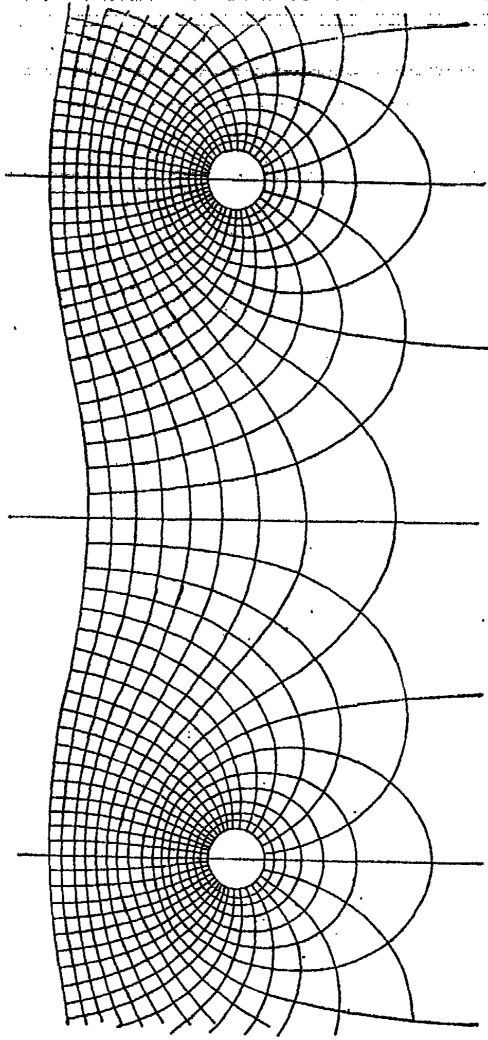
Lignes de force près d'un grillage.
