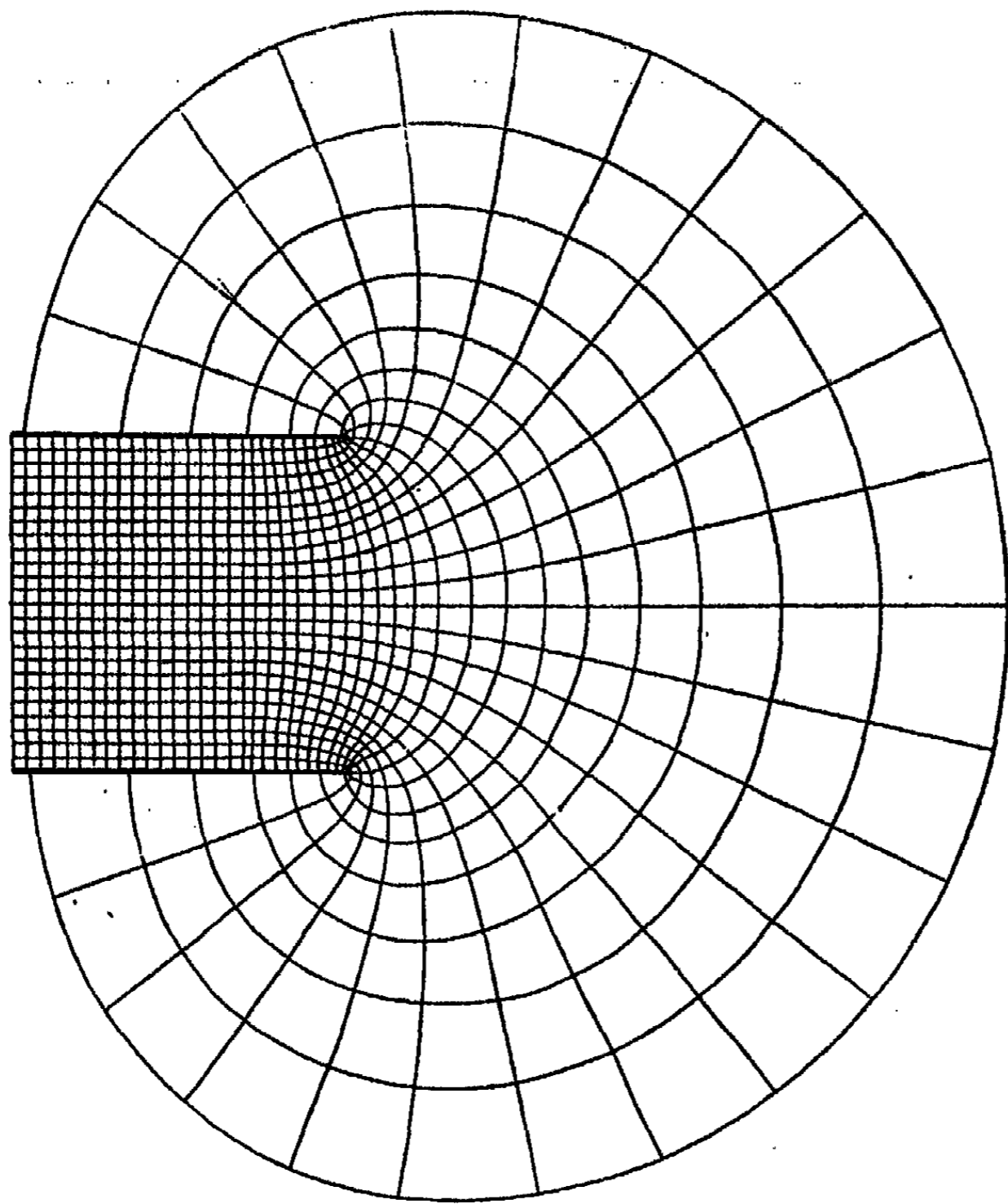
Lignes de force entre deux plaques.
