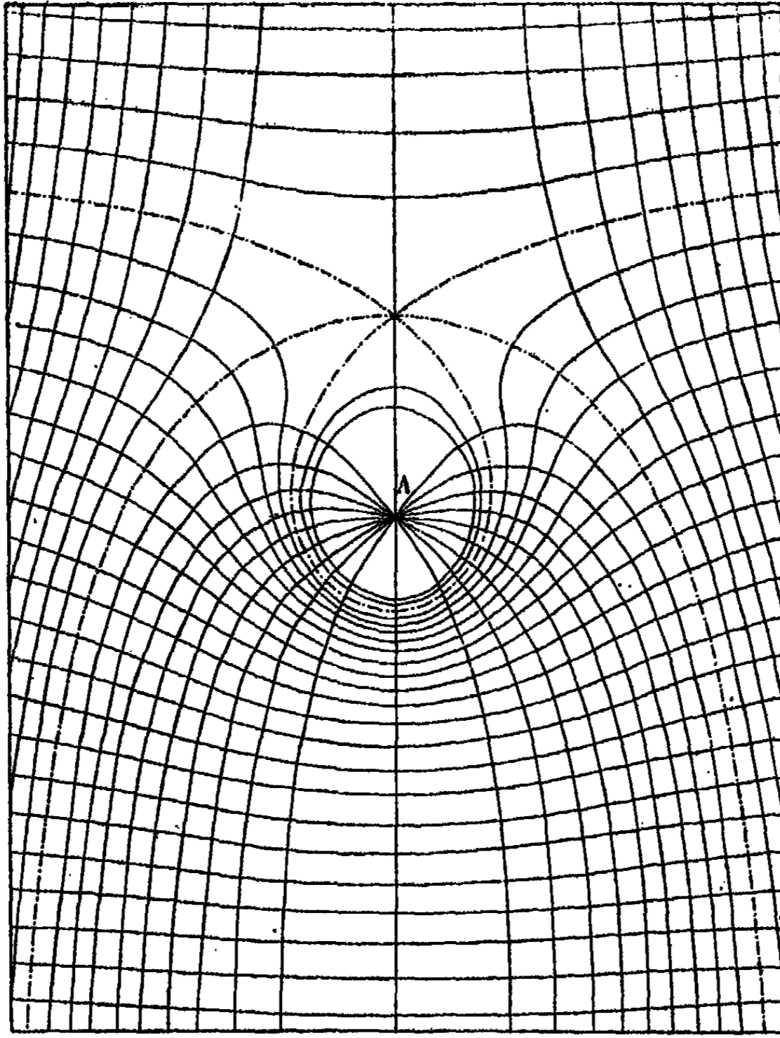
Lignes de force et surfaces équipotentielles.
