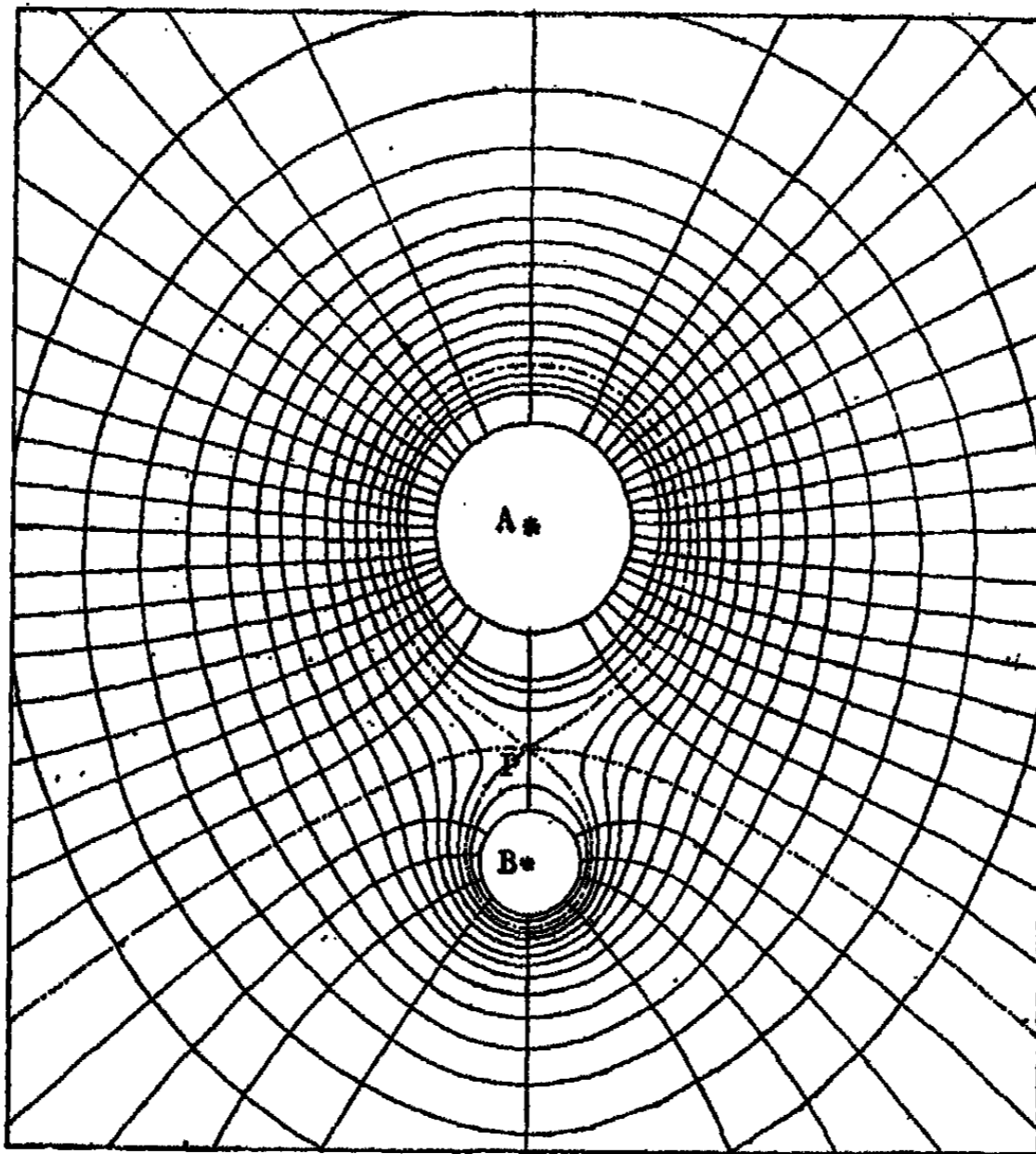
Lignes de force et surfaces équipotentielles.
