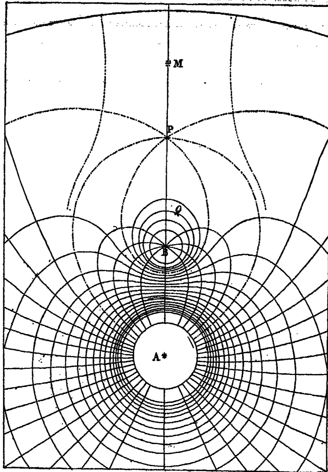
Lignes de force et surfaces équipotentiels.
