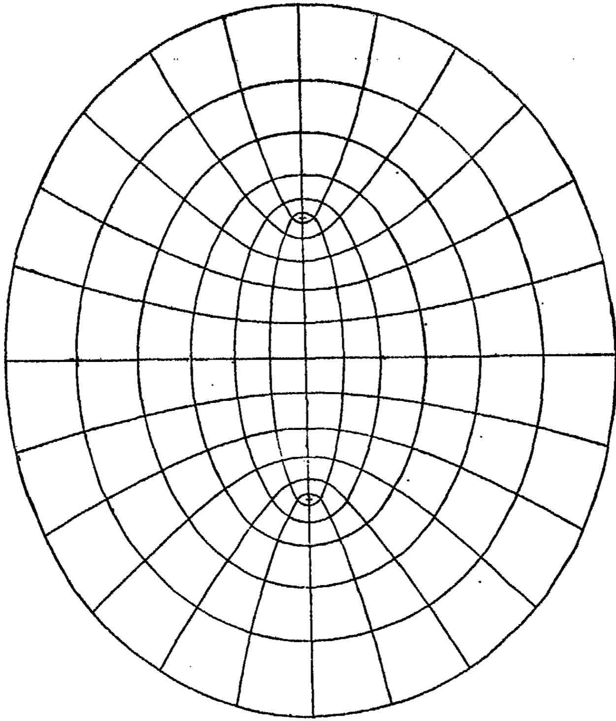
Ellipses et hyperboles confocales.
