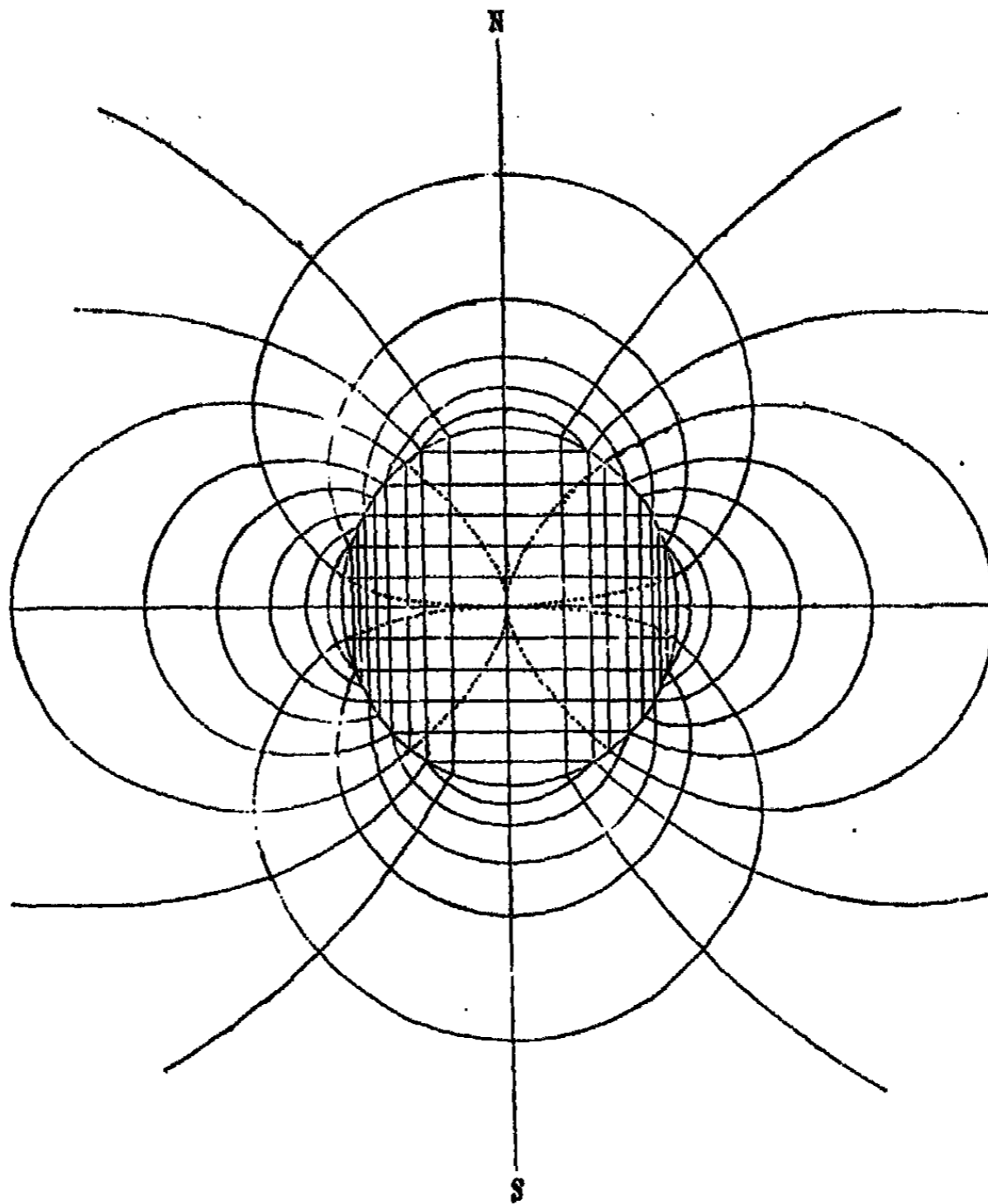
Lignes de force et surfaces équipotentielles dans une section diamétrale d'une surface sphérique, pour laquelle la densité superficielle est un harmonique du premier degré.
