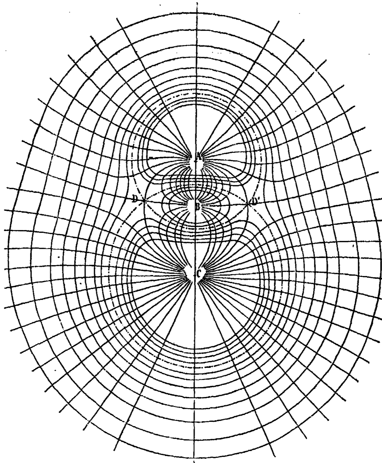
Lignes de force et surfaces équipotentiels.
