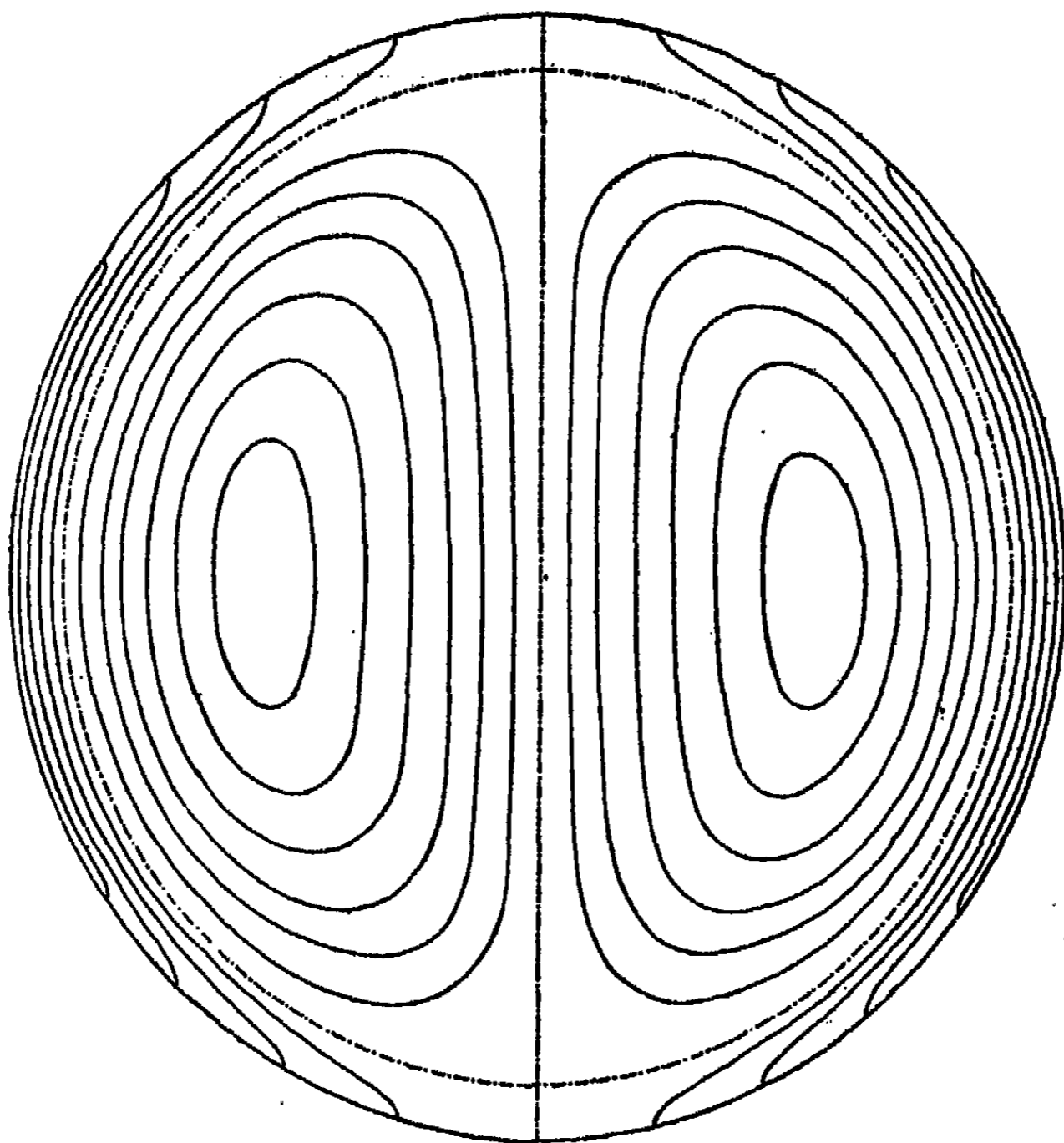
Harmonique sphérique du troisième ordre.
