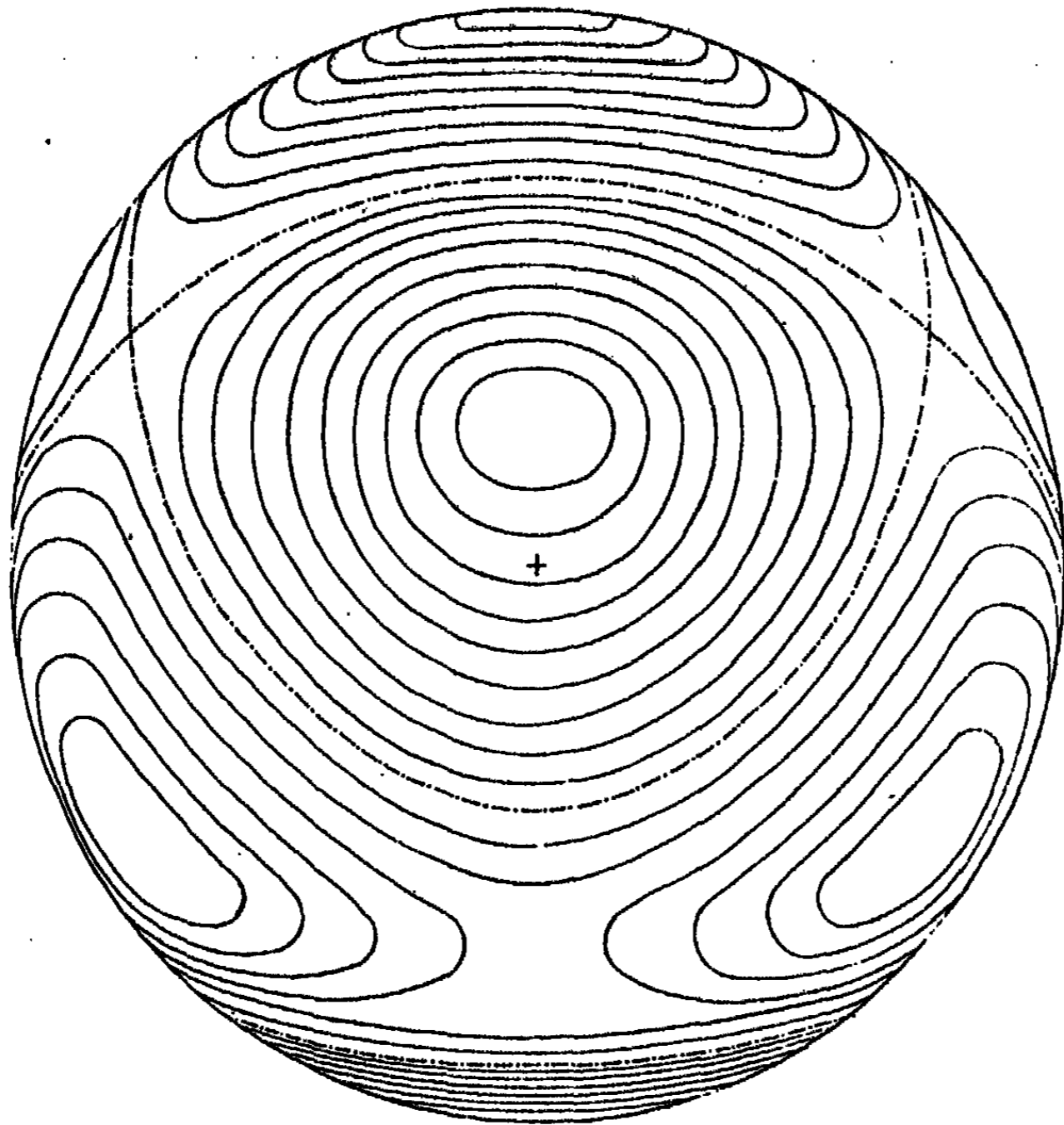
Harmonique sphérique du troisième ordre.
