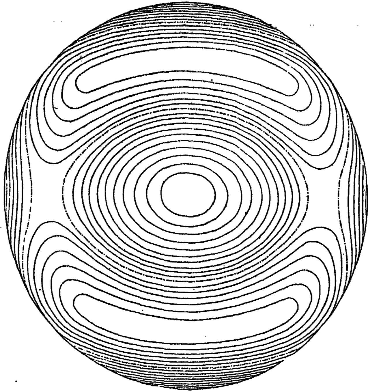
Harmonique sphérique du quatrième ordre.
