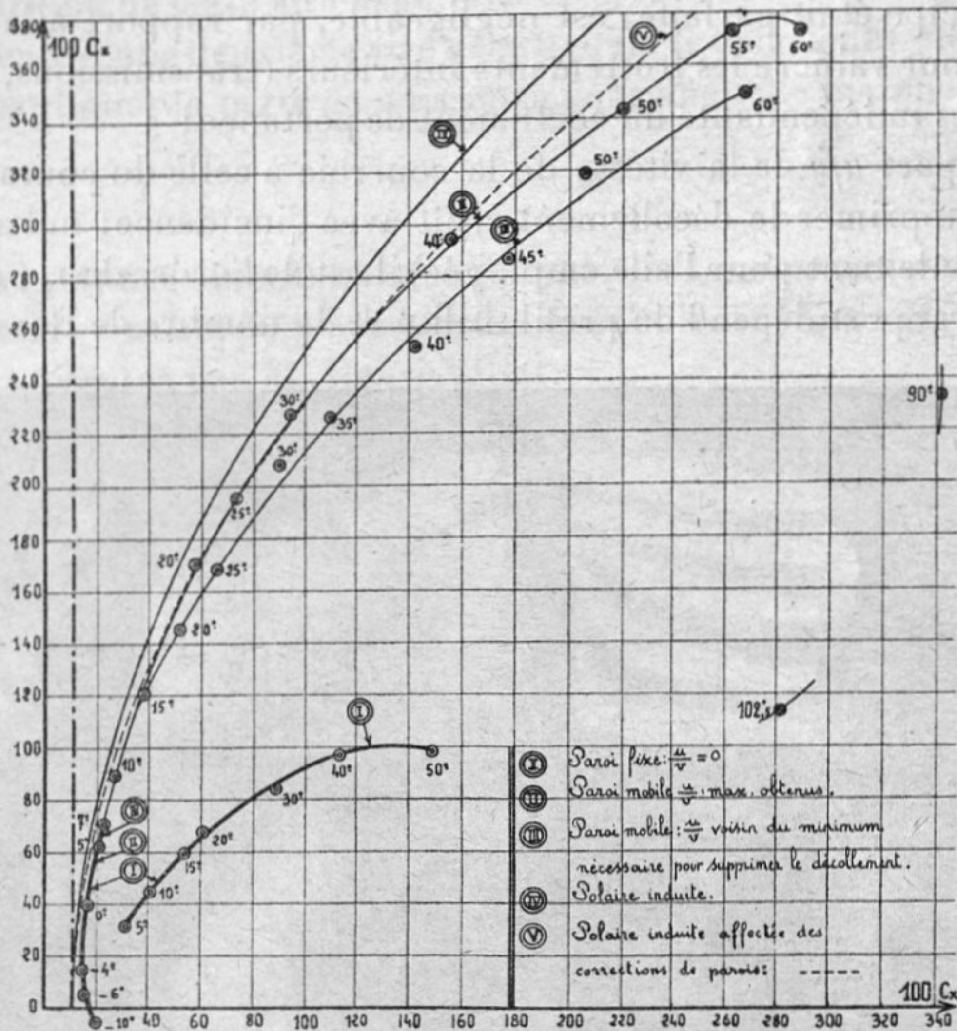
Fig. 2. — Polaire de l'aile à paroi d'extrados mobile; résultats d'ensemble.
